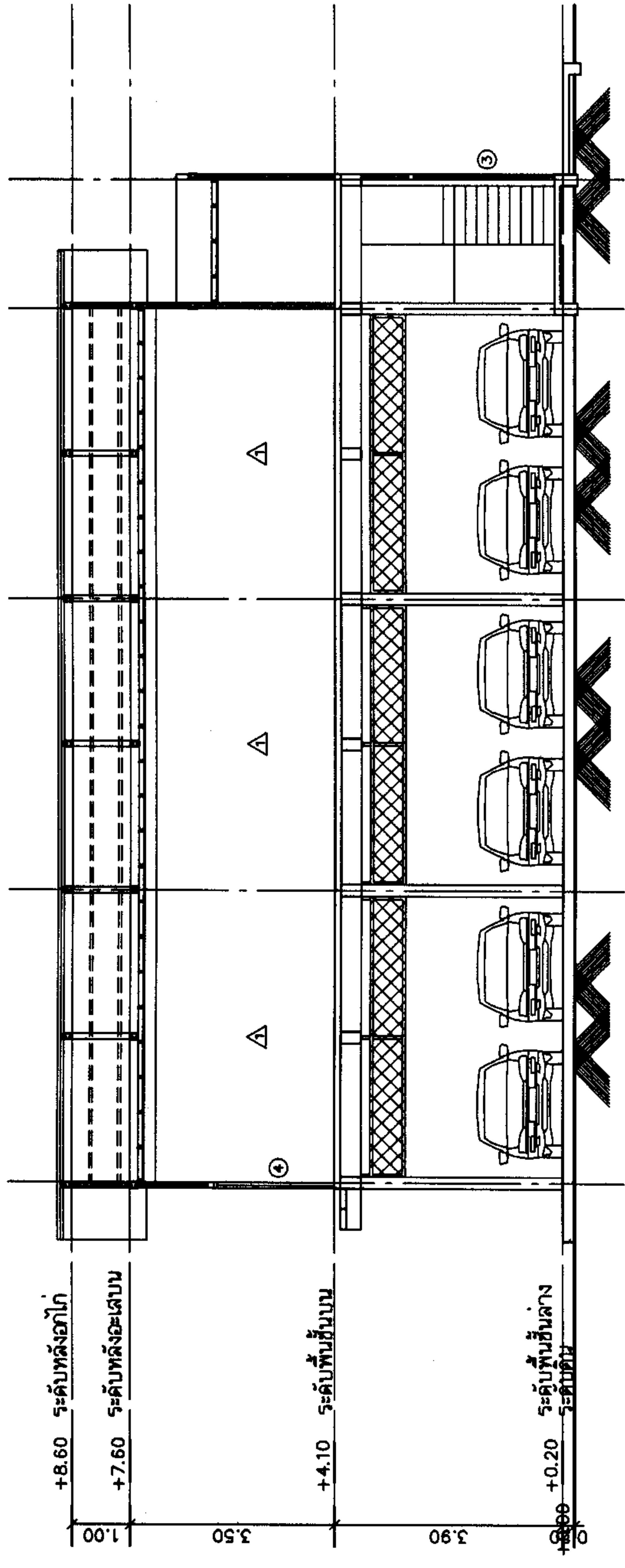
รูปตัด A มาตราส่วน 1 : 100
