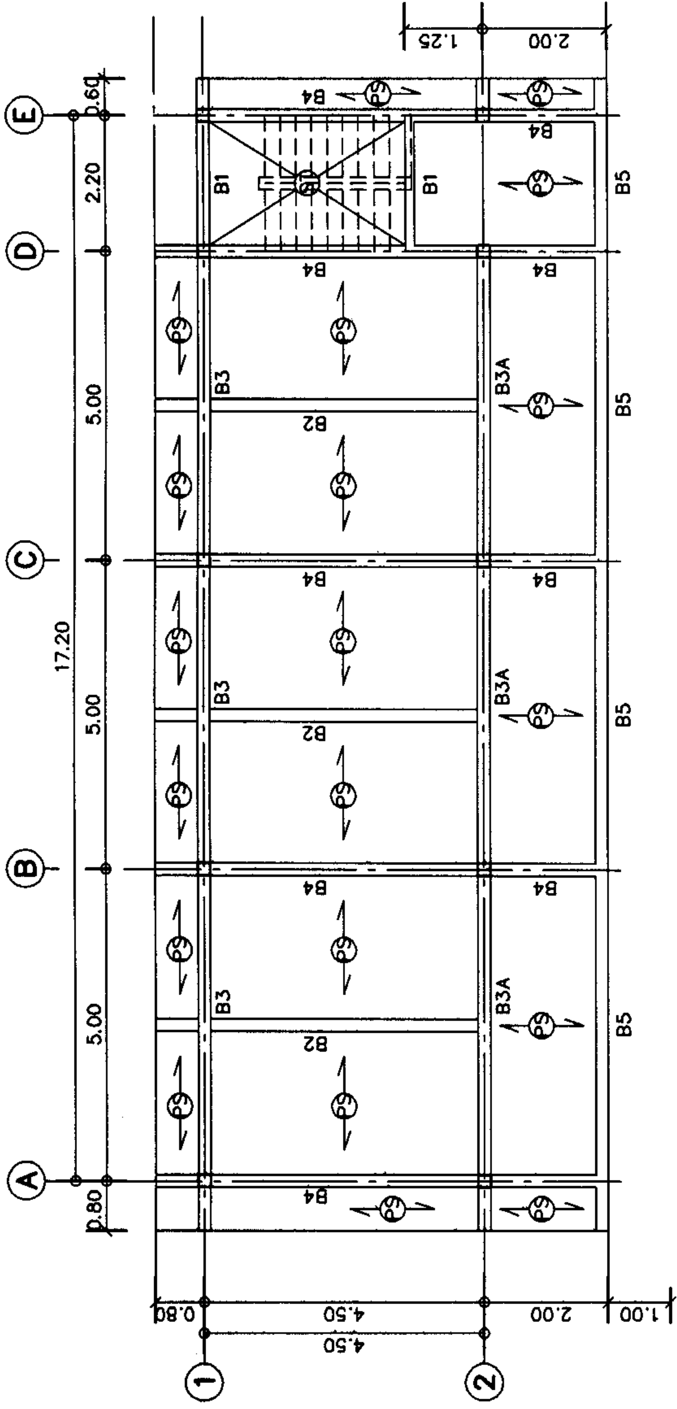
แปลนคานชั้นบน
